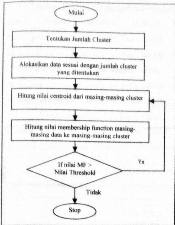
Gambar 1. Algoritma C-Means
